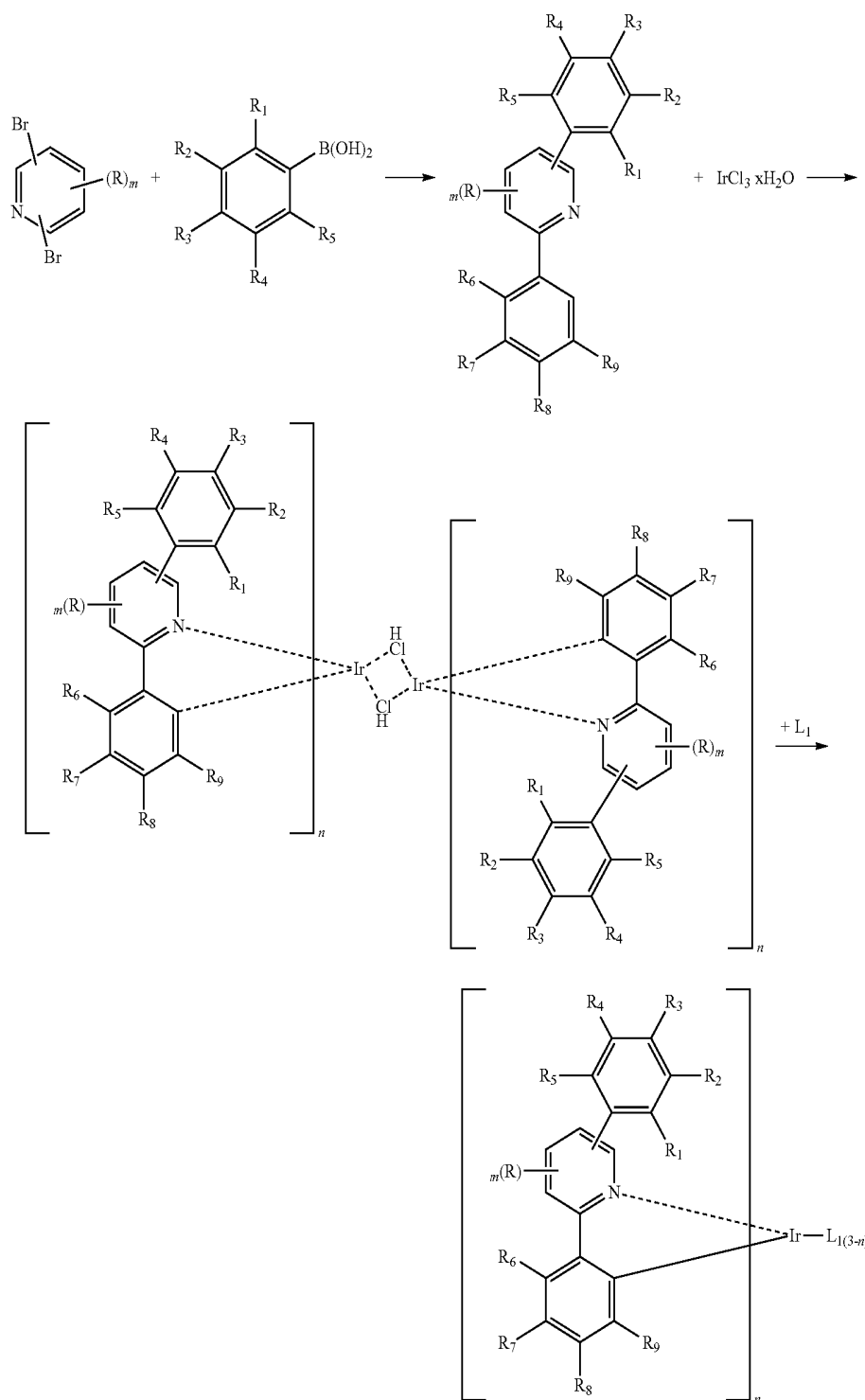
[Scheme 1]
